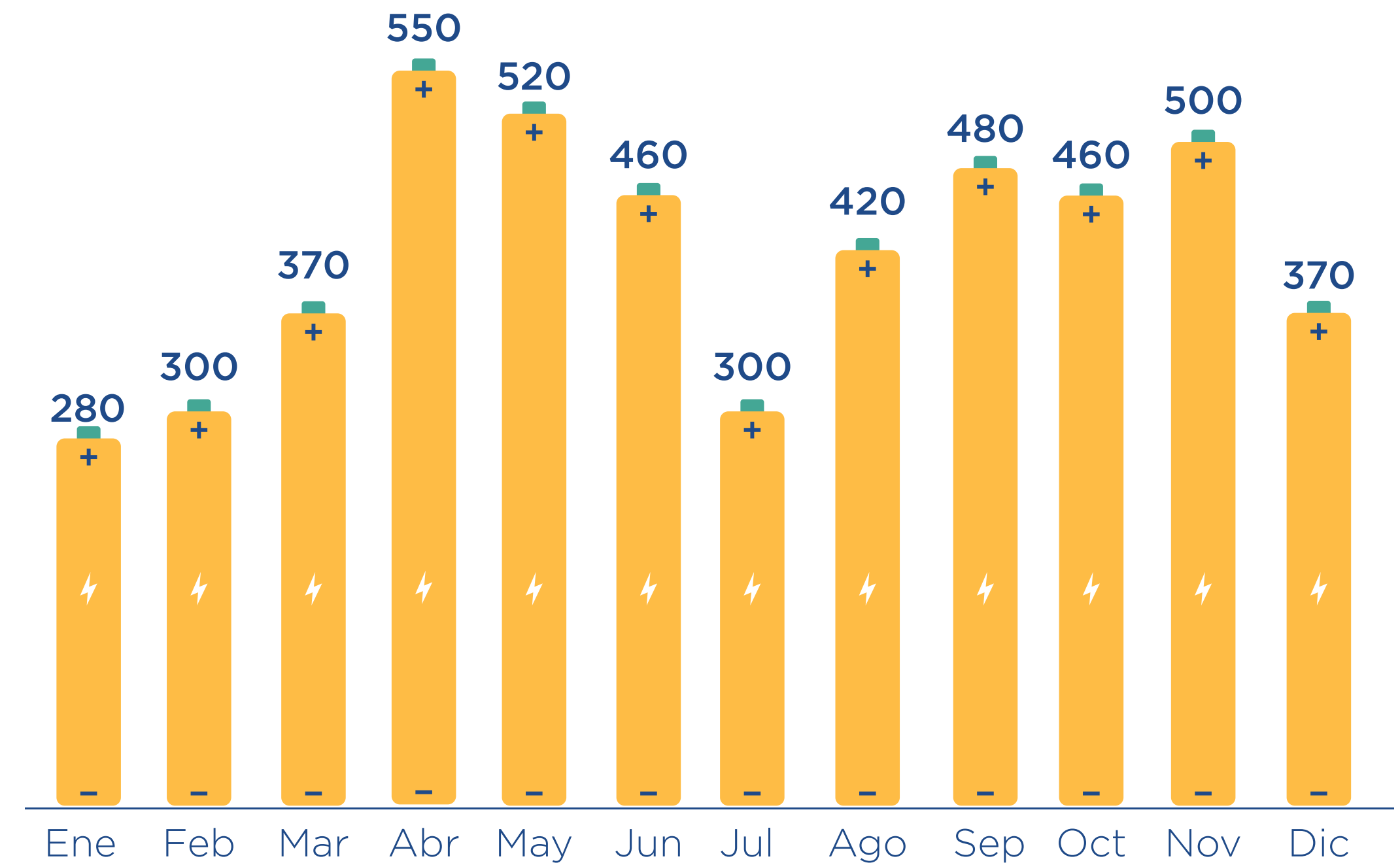
Figura 11: Consumo de energía mensual de la escuela dado por la cuenta de energía eléctrica.
