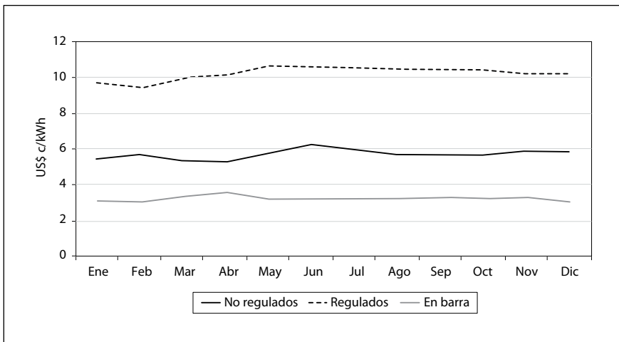
GRÁFICO 1 Precios regulados, en barra y no regulados
