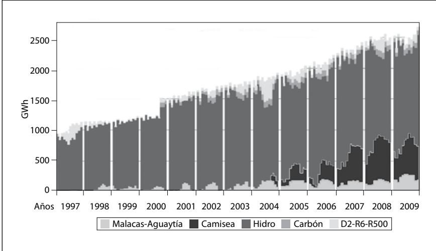
GRÁFICO 2 Evolución de la producción de energía del SEIN por tipo de generación (GWh)
