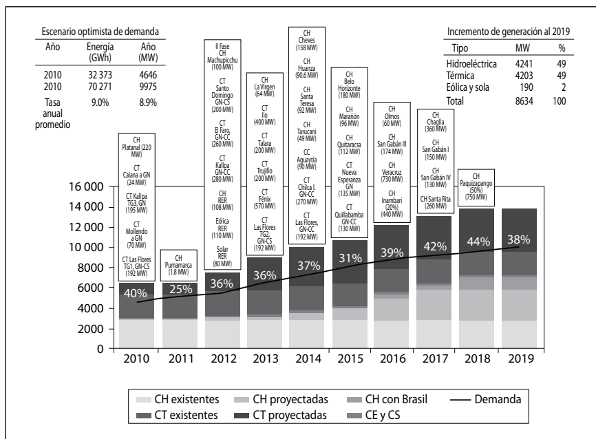
GRÁFICO 5 Balance eléctrico de potencia-demanda del SEIN 2010-19
