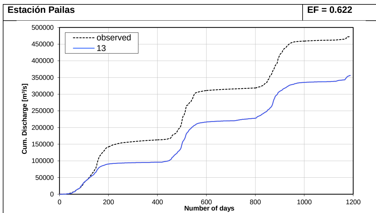
Figura 106. Acumulados de Caudal Observados y Modelados
