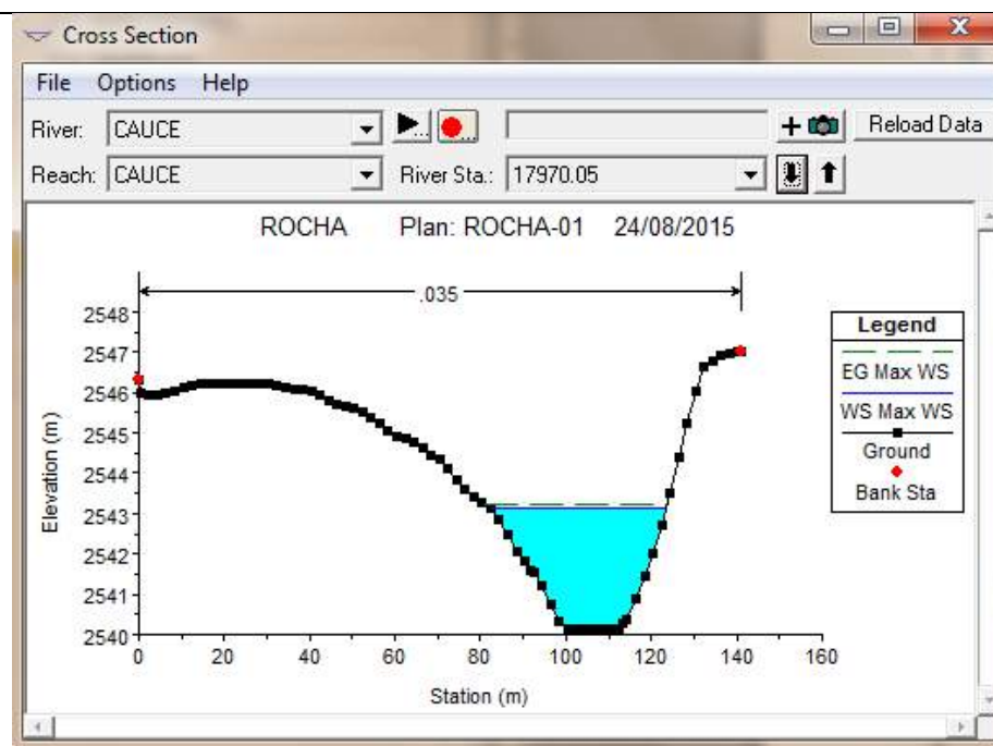
Figura 118. a) Curva de Descarga Puente Cajon (Aeropuerto-CBBA) vs. Sección 17970.05 y b) Sección 17970.05 (HEC-RAS)
