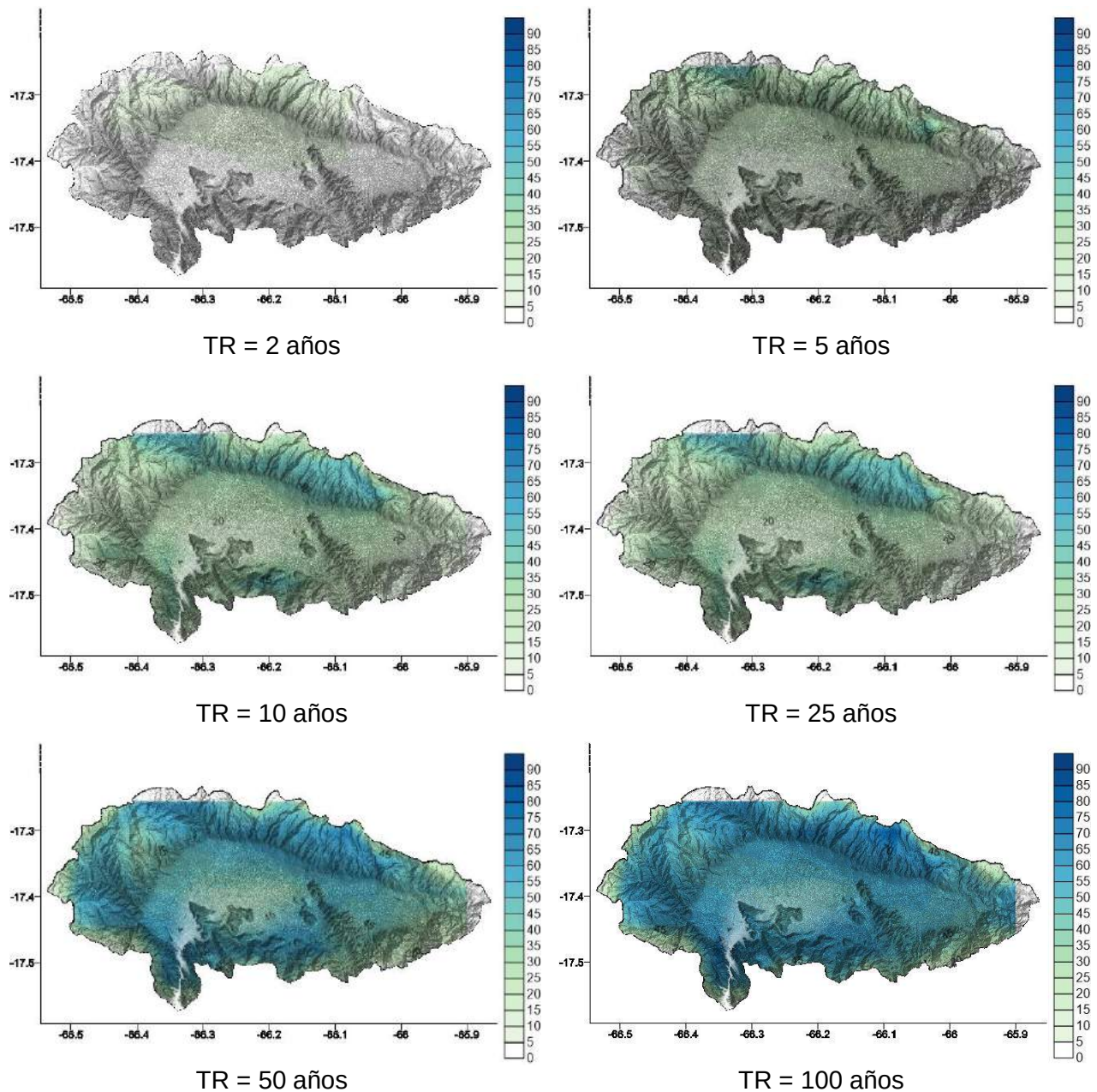
Figura 79. Distribución de amenaza probabilista de lluvias – Duración: 1 día - Cuenca del río Rocha. Profundidad de precipitación en [mm]
