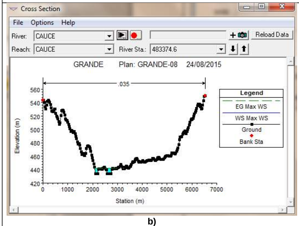
Figura 120. a) Curva de Descarga Abapó (Paraíso) vs. Sección 483374.6 y b) Sección 483374.6 (HEC-RAS)
