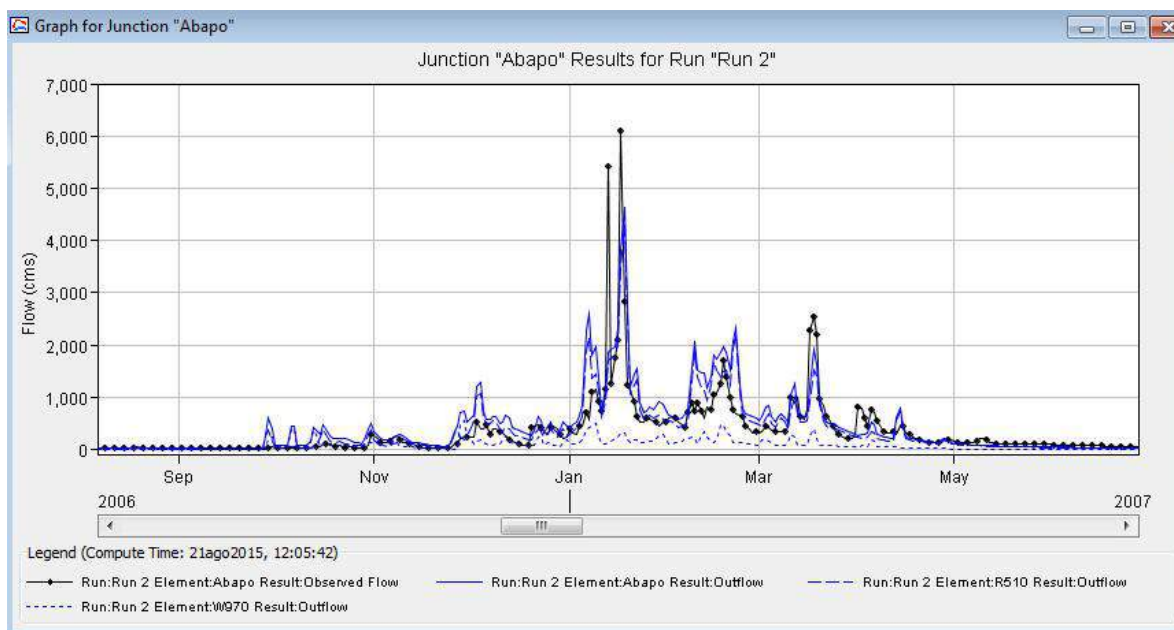
Figura 103. Corrida en HEC-HMS para un año (2006-2007), Estación Abapó
