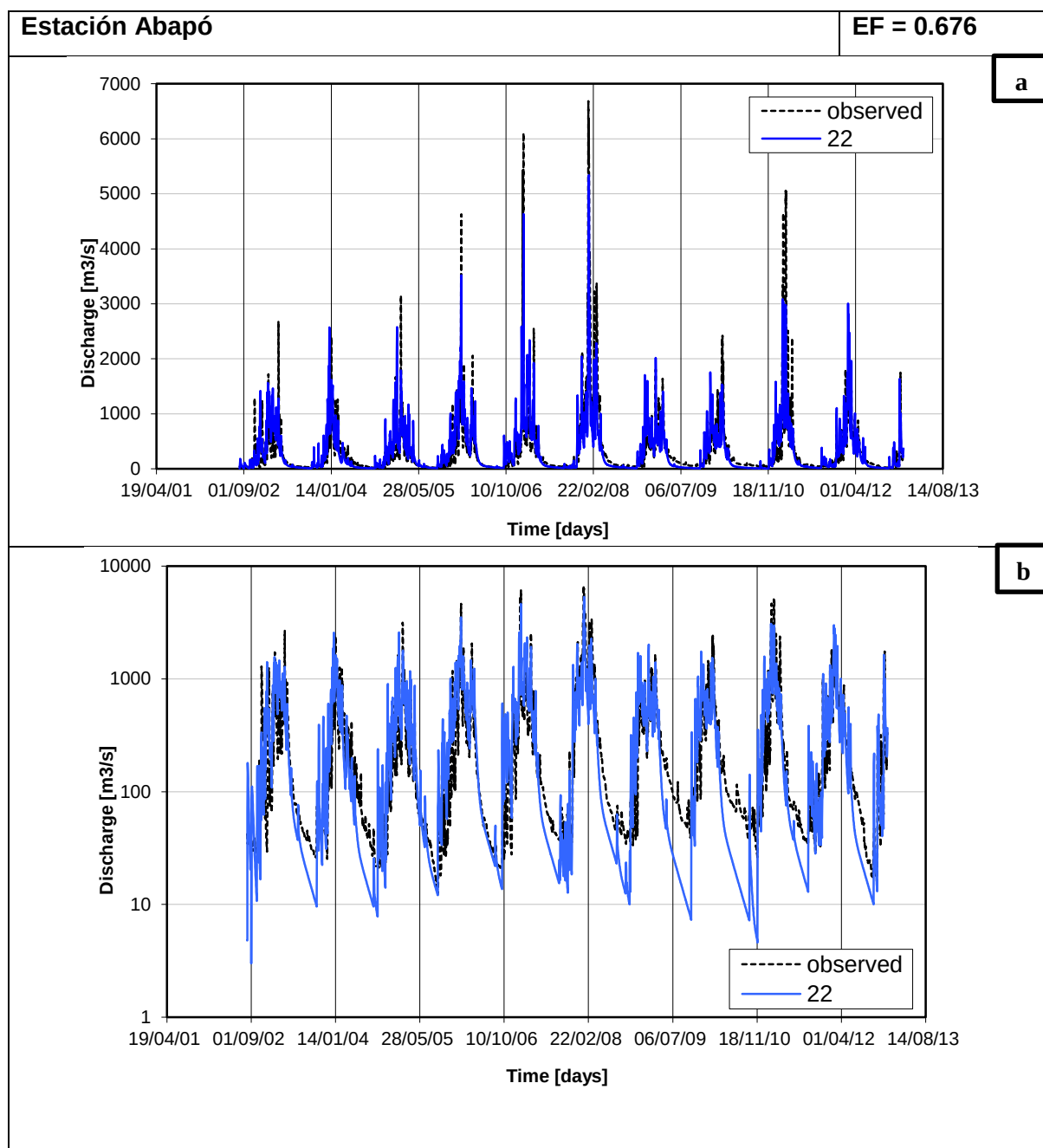
Figura 99. Serie de tiempo de caudales Observados y Modelados: a) Escala Lineal y b) Escala Semi-logarítmica
