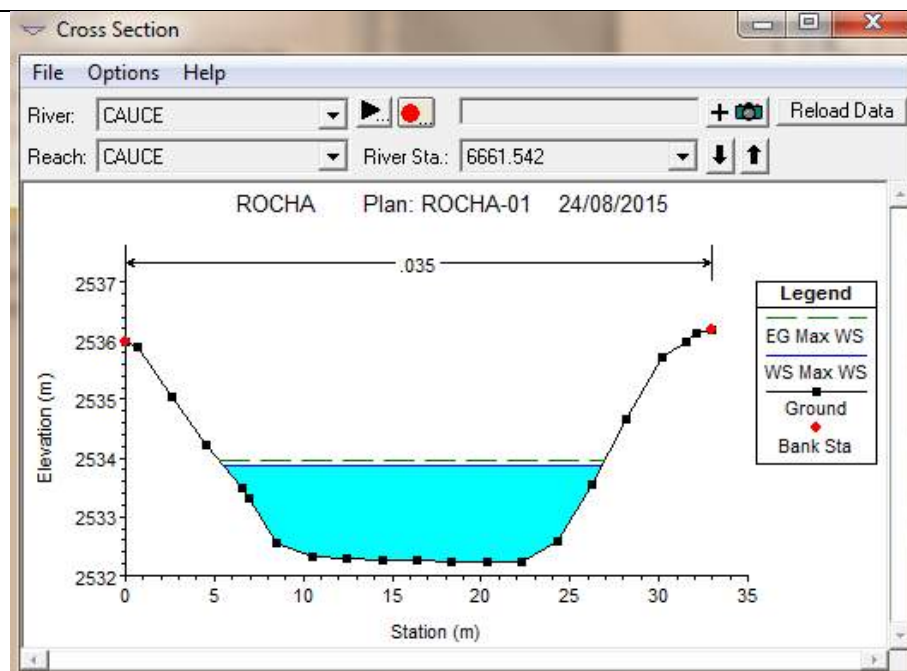
Figura 119. a) Curva de Descarga Puente Urkupiña vs. Sección 6661.542 extendida y b) Sección 6661.542 (HEC-RAS)
