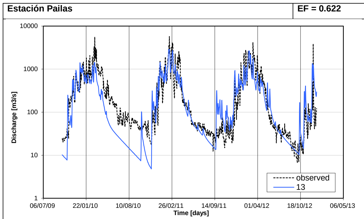
Figura 105. Serie de tiempo de caudales Observados y Modelados (Escala Semi-logarítmica)
