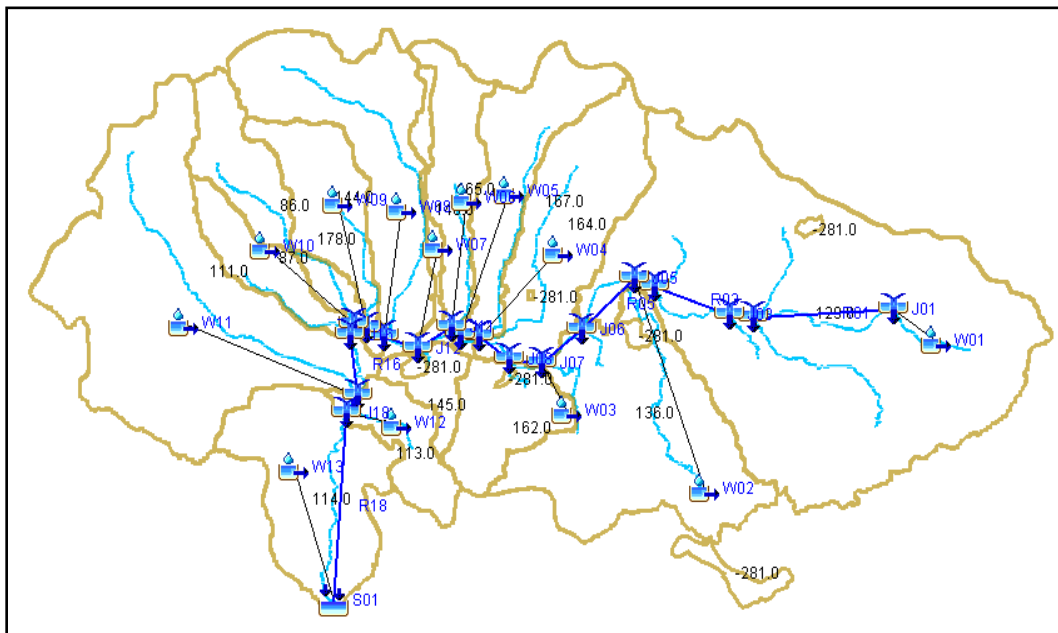
Figura 89. Representación del sistema de la cuenca del río Rocha en el software HEC – HMS
