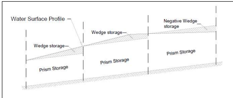
Figura 90. Gráfica de almacenamiento de cuña.
