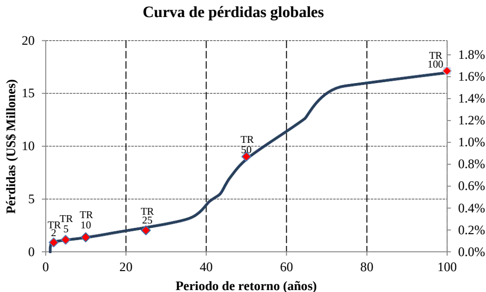
Figura 143. Curva de pérdida máxima probable vs. periodo de retorno. Cuenca Río Rocha
