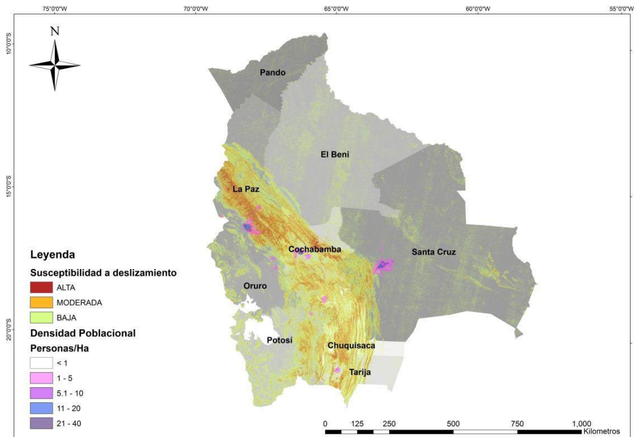
Figura 51. Resultados típicos de análisis de susceptibilidad a los deslizamientos condición 2.
