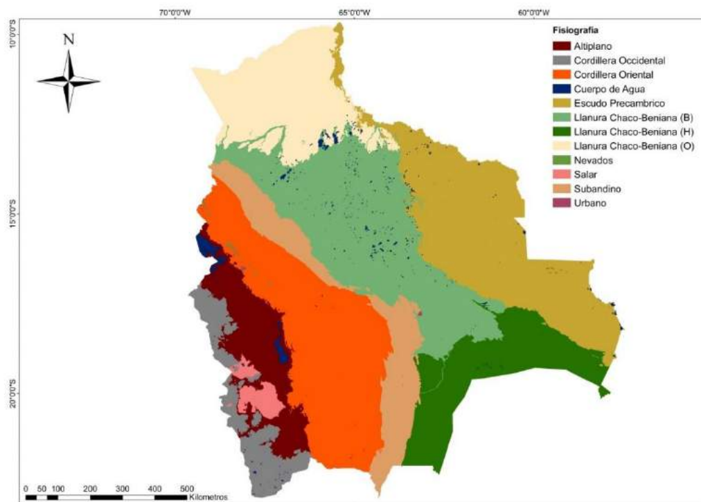
Figura 28. Fisiografía.
