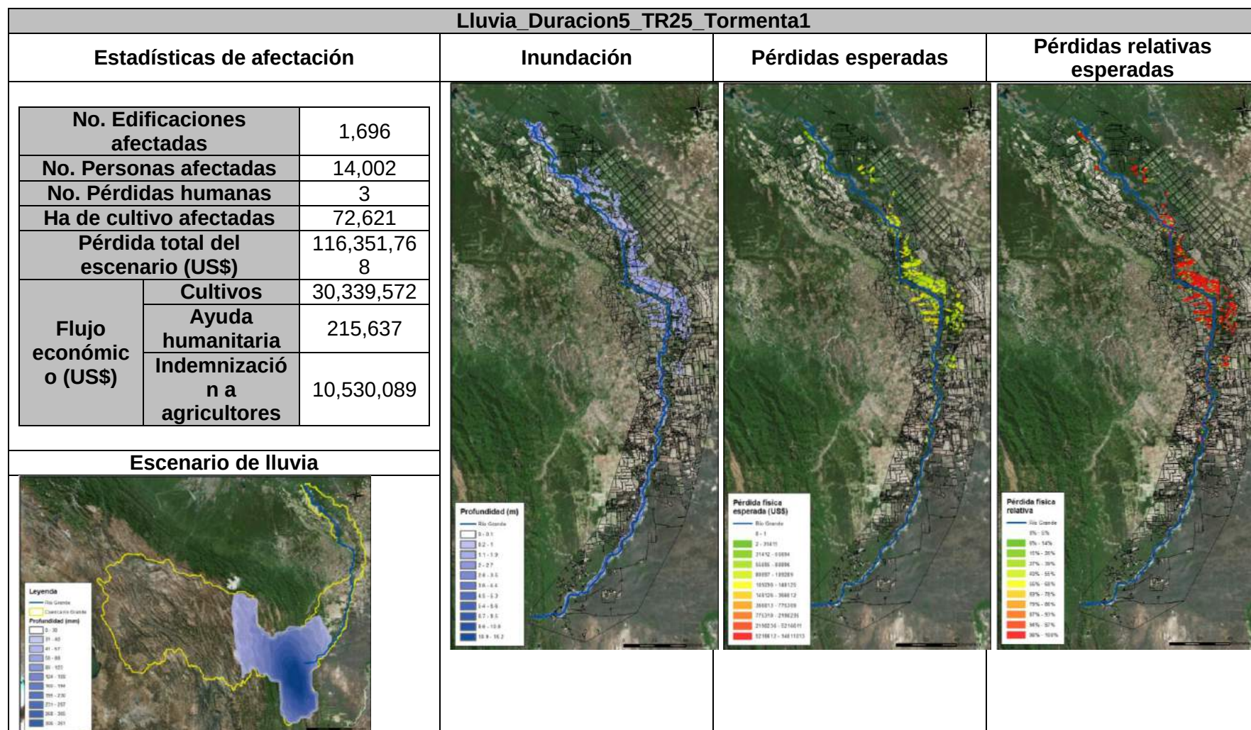
Figura 163. Resultados para el escenario 11. Cuenca Río Grande
