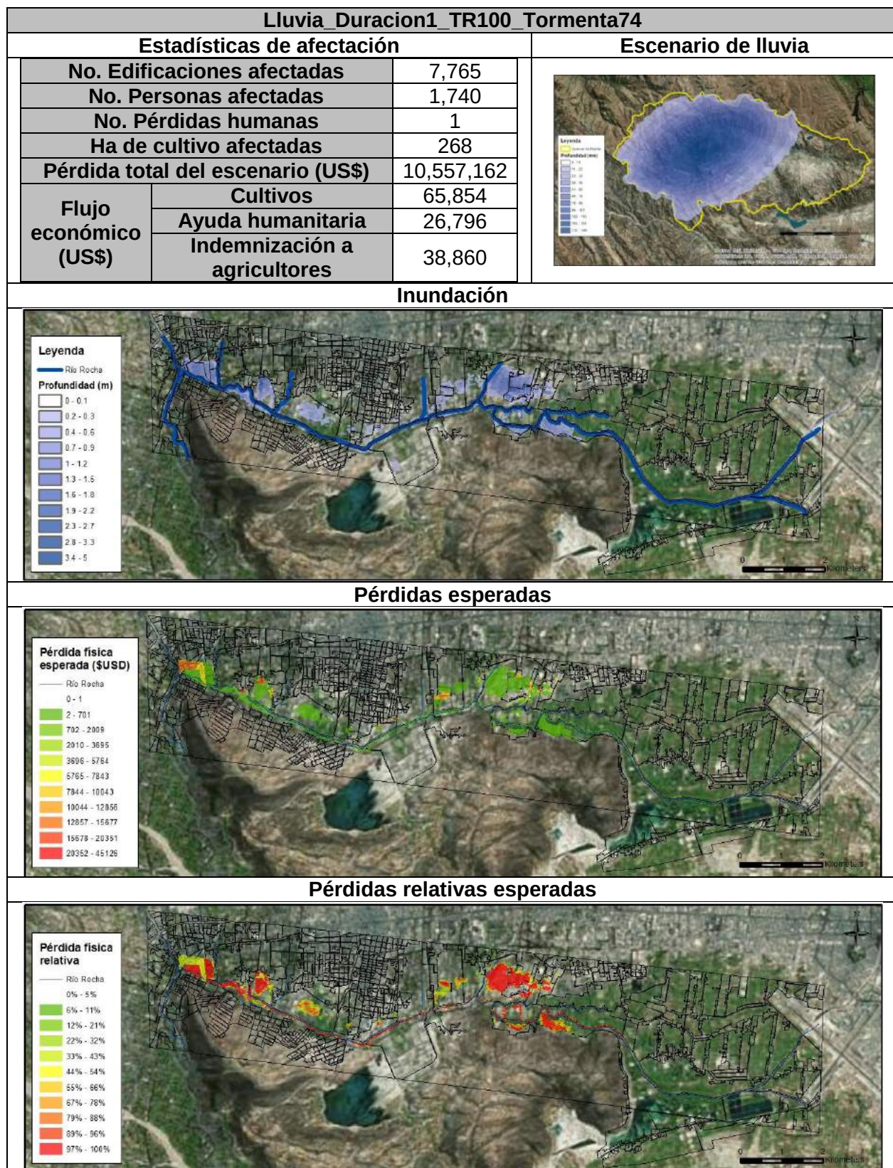
Figura 151. Resultados para el escenario 575. Cuenca Río Rocha
