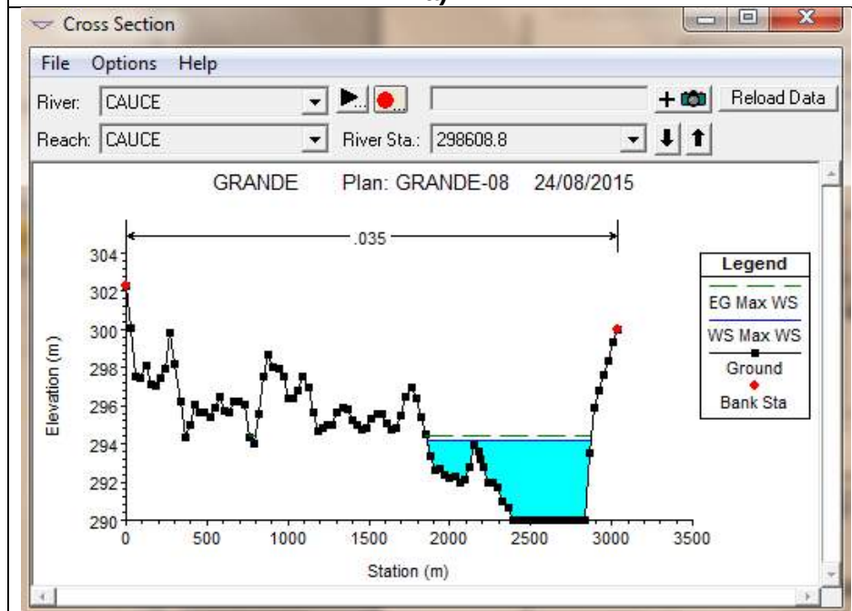
Figura 121. a) Curva de Descarga Puente Pailas vs. Sección 298608.8 y b) Sección 298608.8 (HEC-RAS)
