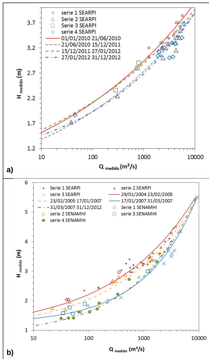
Figura 111. Variación temporal de la curva de descarga: a) Puente Pailas periodo 2010 – 2012, b) Abapó periodo 2005 - 2012
