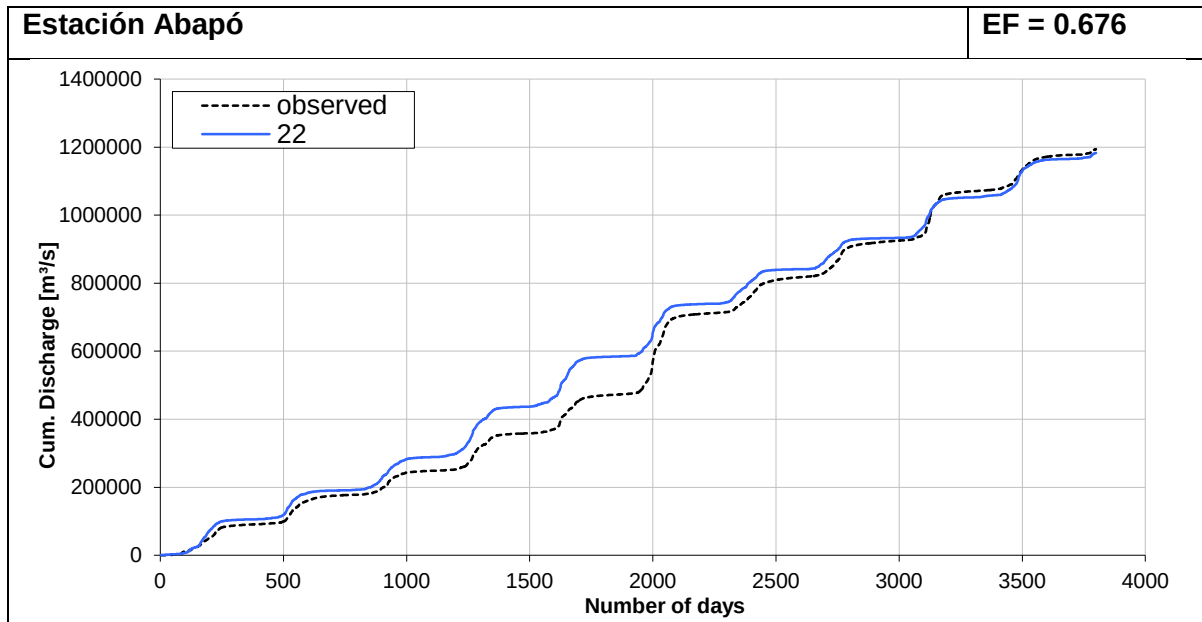
Figura 100. Acumulados de Caudal Observados y Modelados
