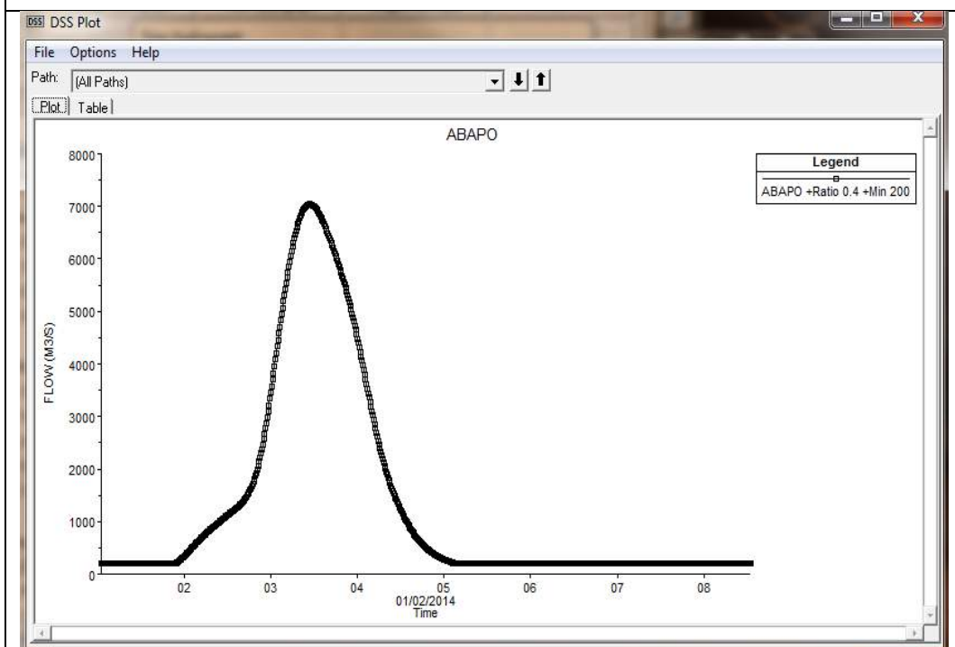
Figura 116. Hidrogramas de entrada al modelo HEC-RAS: a) Rio Rocha y b) Rio Grande
