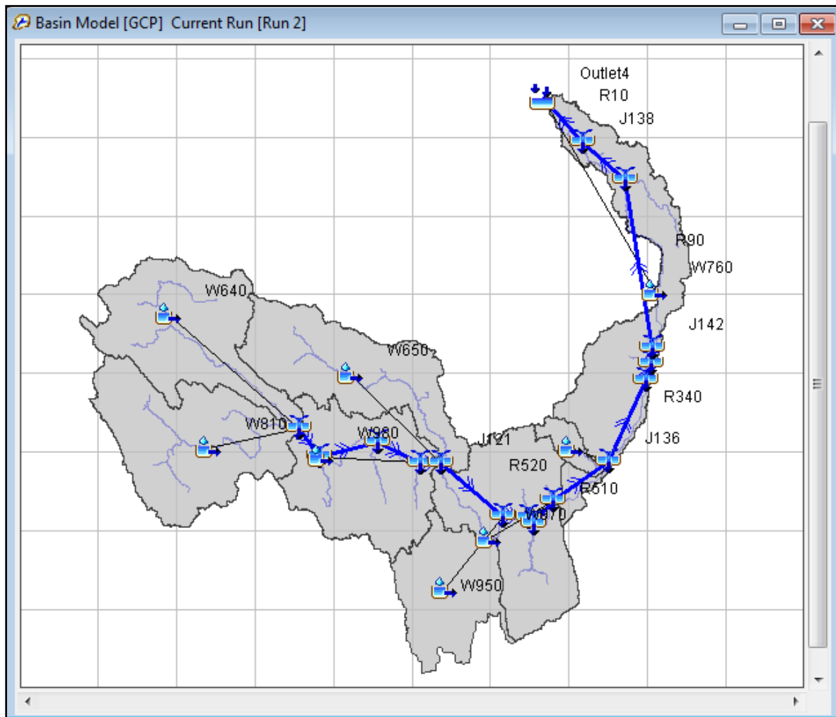
Figura 98. Esquema de la Cuenca del Río Grande cargado al HEC – HMS
