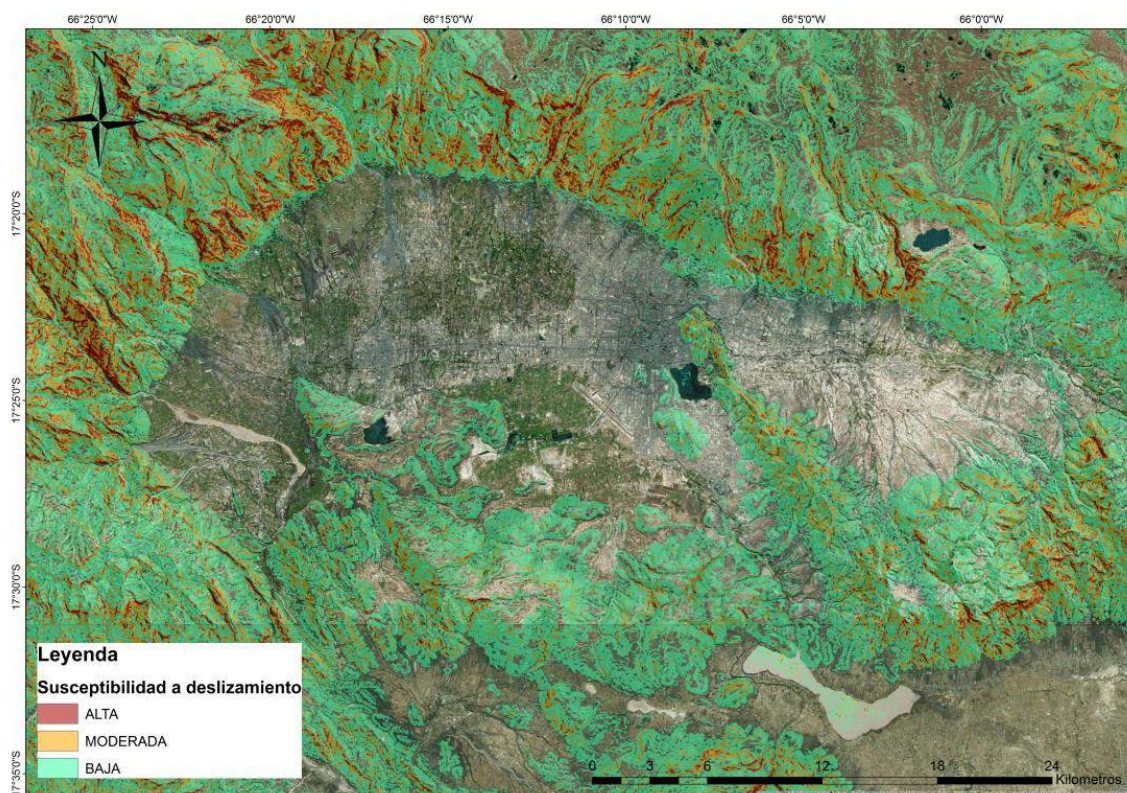
Figura 56. Resultados típicos de análisis de susceptibilidad a los deslizamientos condición 2, ciudad de Cochabamba.
