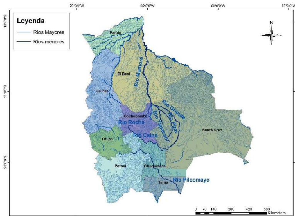
Figura 63. Ríos principales.
