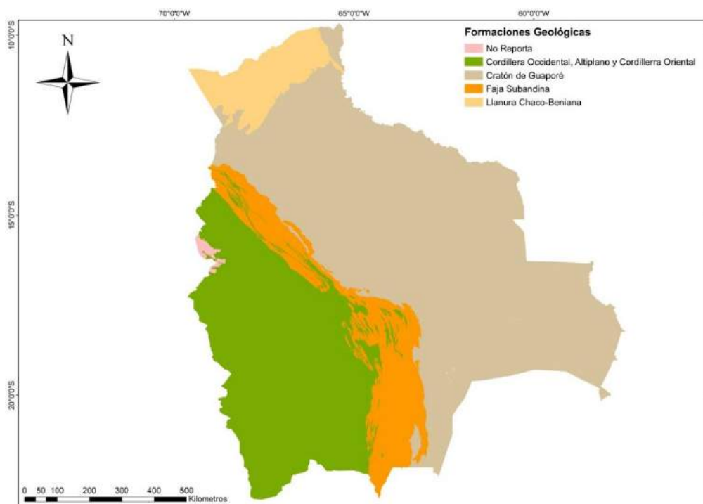
Figura 27. Formaciones geológicas.
