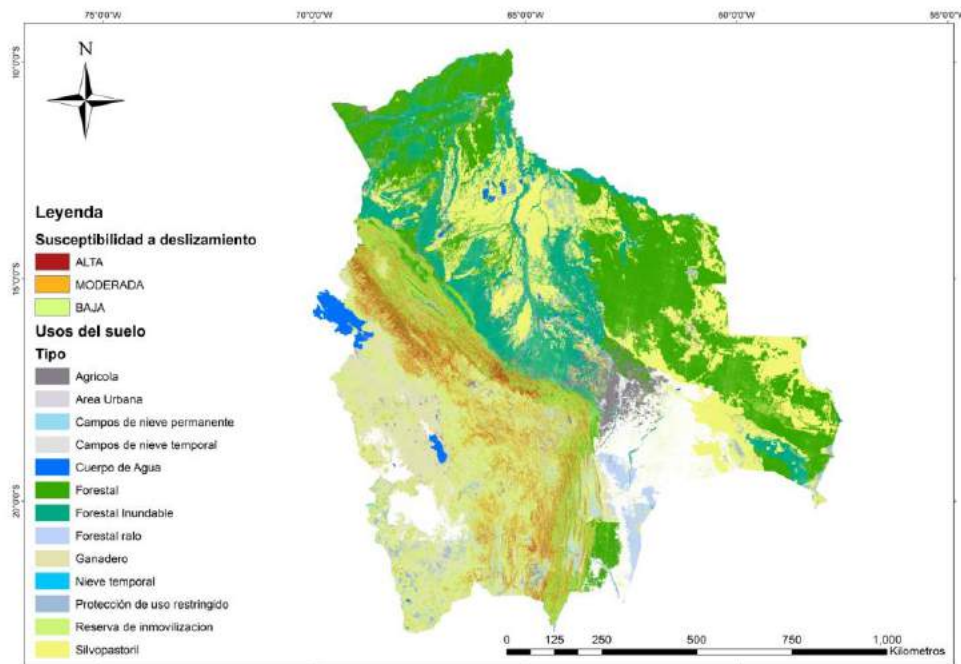
Figura 61. Zonas susceptibles a deslizamientos según uso del suelo para la condición 2 de análisis.
