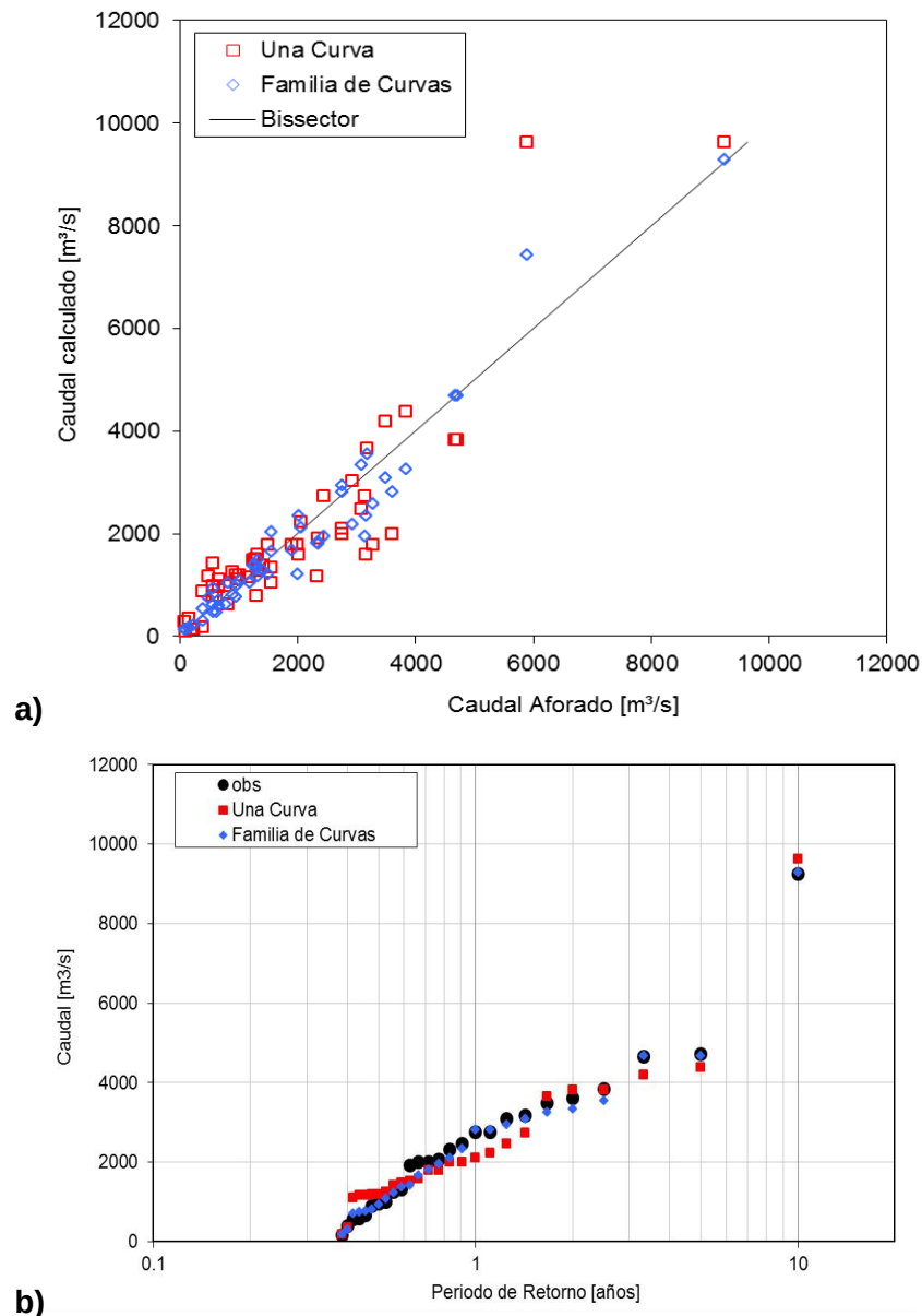
Figura 112. Comparación de las técnicas de Familia de curvas de descarga vs. una sola curva, estación Abapó: a) grafica de dispersión, b) distribución empírica de valores extremos
