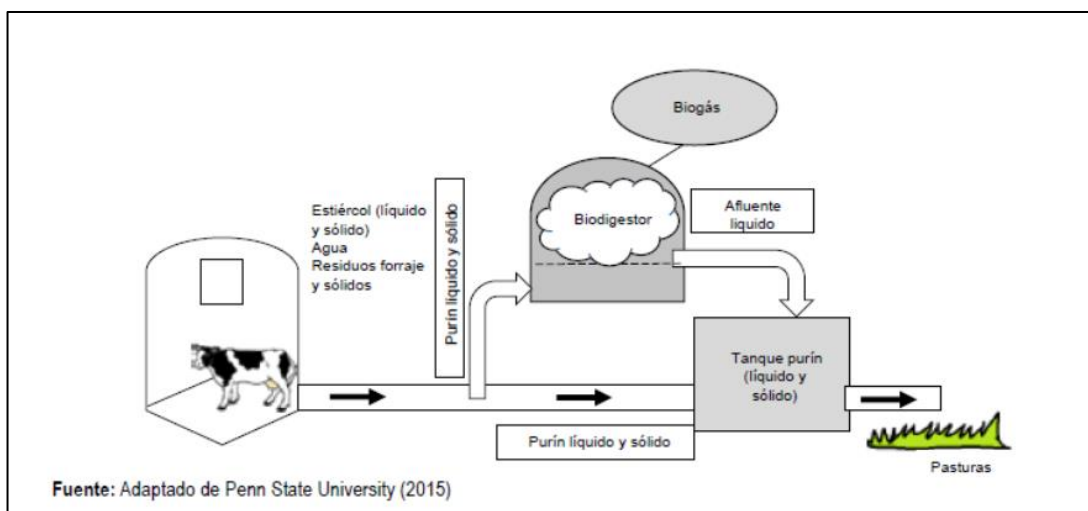
Figura 15. Sistema de gestión de excretas sólidas y líquidas con inclusión de un biodigestor (Fuente: Lombo et al. 2015).
