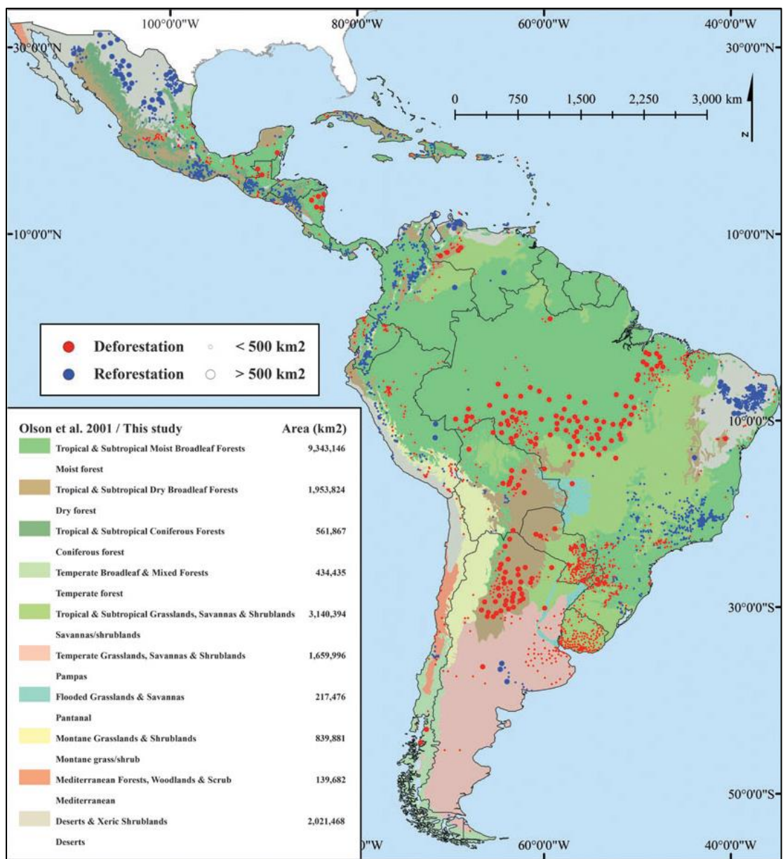
Figura 2 Distribución de las áreas críticas de deforestación y reforestación en los principales biomas en LAC, entre el 2001 y el 2010 (Aide et al. 2013)
