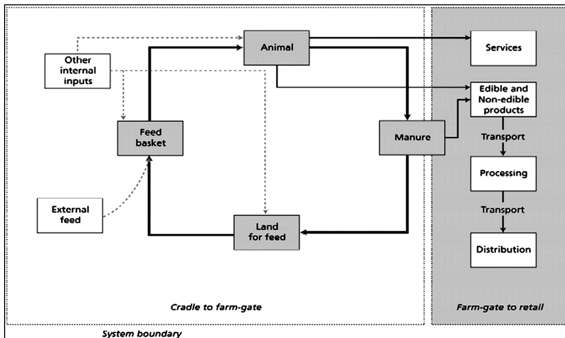
Figura 12. Límites del sistema para el ACV en el sector lechero (Gerber et al. 2011).
