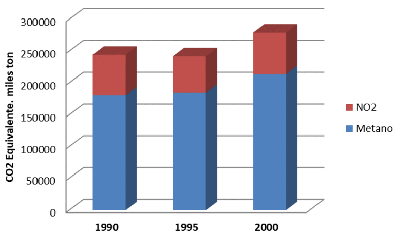
Figura 3. Emisión de metano y óxido nítrico por los sistemas de producción agropecuaria en América Central, para el período 1990 - 2000 (Pezo et al. 2012b).
