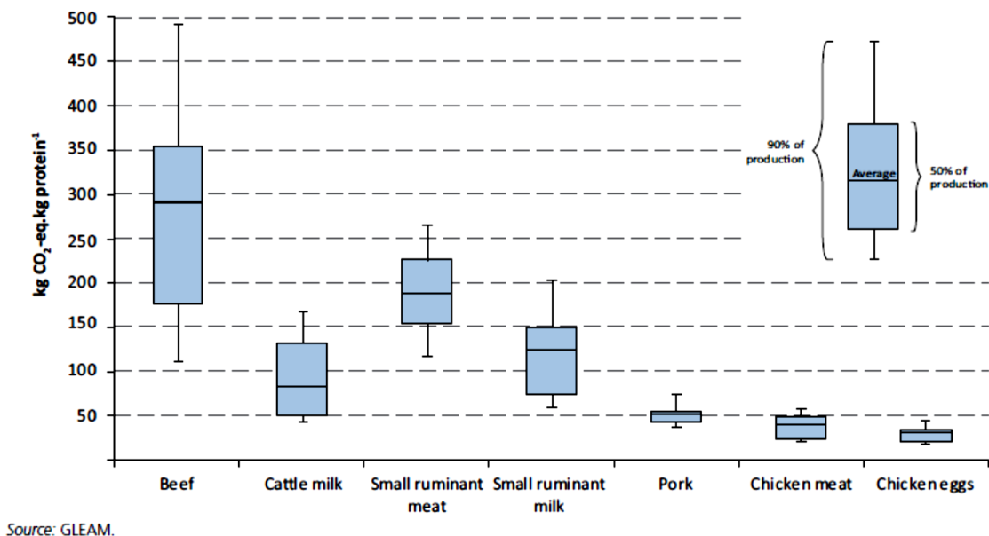
Figura 7. Intensidad de emisiones de GEI (kg de CO 2 equiv por kg de proteína) para diferentes rubros de origen animal (Gerber et al. 2013c).
