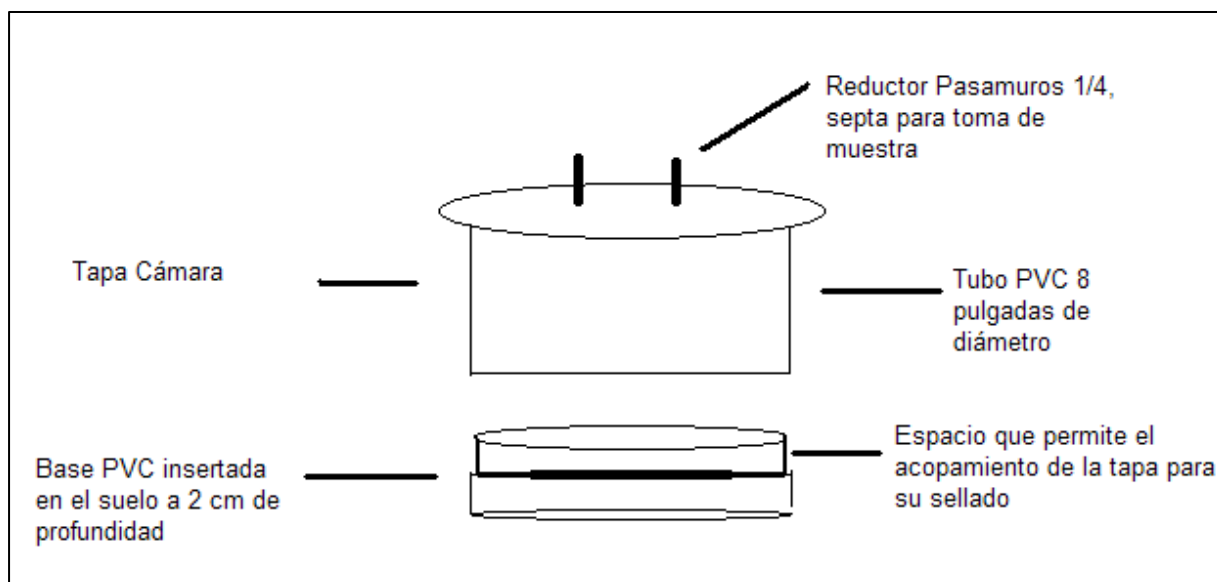
Figura 10. Diseño de una cámara de muestreo de GEI en el suelo (Saldaña-Munive et al. 2014).
