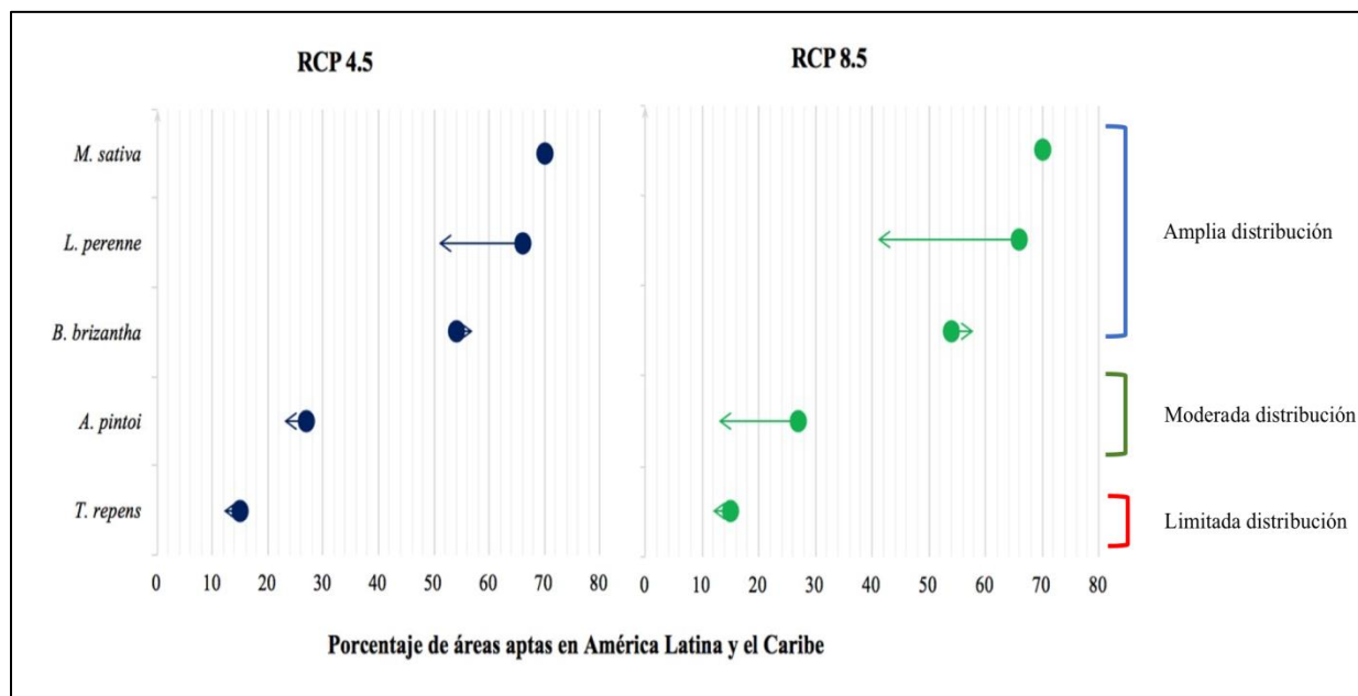
Figura 4 Cambios relativos en las áreas potencialmente aptas para el crecimiento de forrajeras de zona templada y tropical, en función de cambios moderados (RCP 4,5) y extremos (RCP 8,5) en el clima entre el presente y el año 2050.
