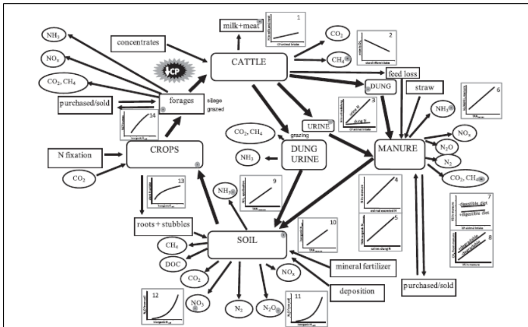
Figura 11. Diagrama conceptual de los componentes, almacenes y flujos de C y N en un sistema ganadero que incluye pastoreo (Del Prado et al 2013)
