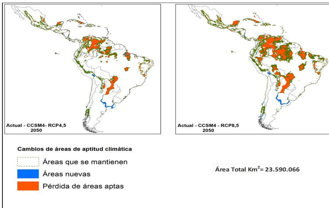
Figura 5. Cambios en la distribución potencial de las áreas aptas para ryegrass ( Lolium perenne ) en América Latina y el Caribe, entre el presente y el año 2050, en función de dos escenarios de cambio climático (RCP 4,5 y 8,5).
