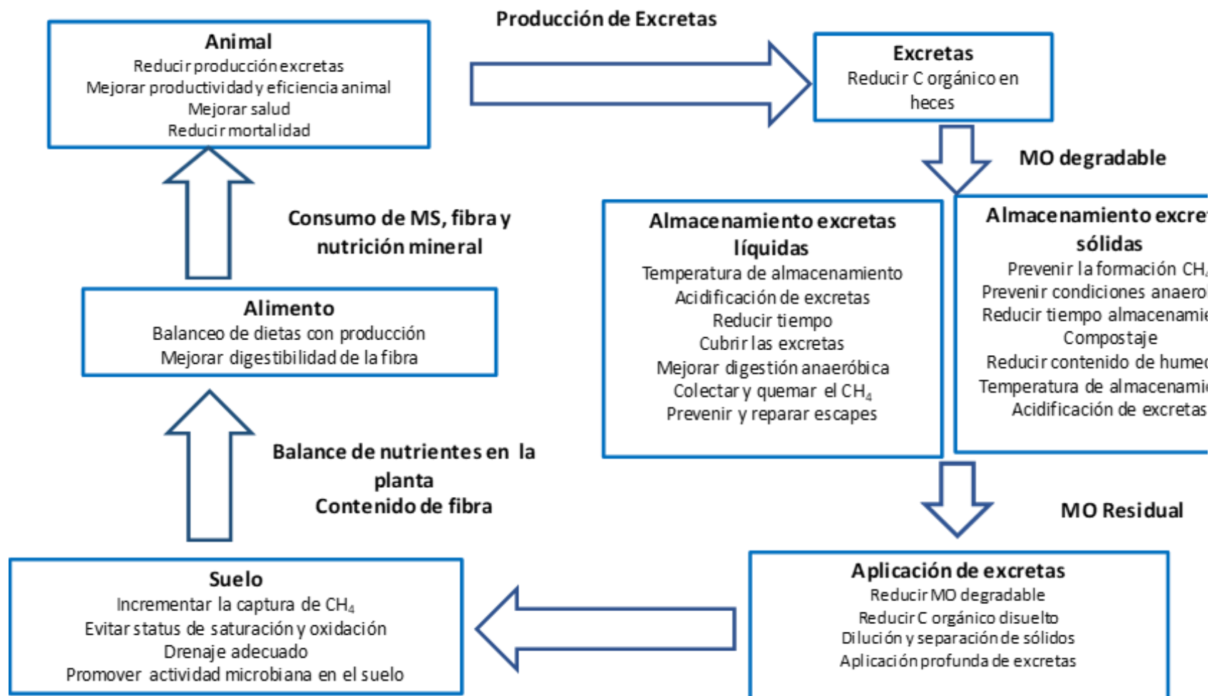
Figura 13. Oportunidades de mitigación de metano a partir de las excretas del ganado (Adaptado de: Montes et al. 2013)
