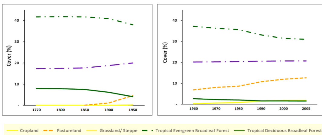
Figura 1. Cambios de uso de la tierra en LAC entre los años 1770 y 2005 (Basado en datos presentados por UI-UC/ATMO, 2018)
