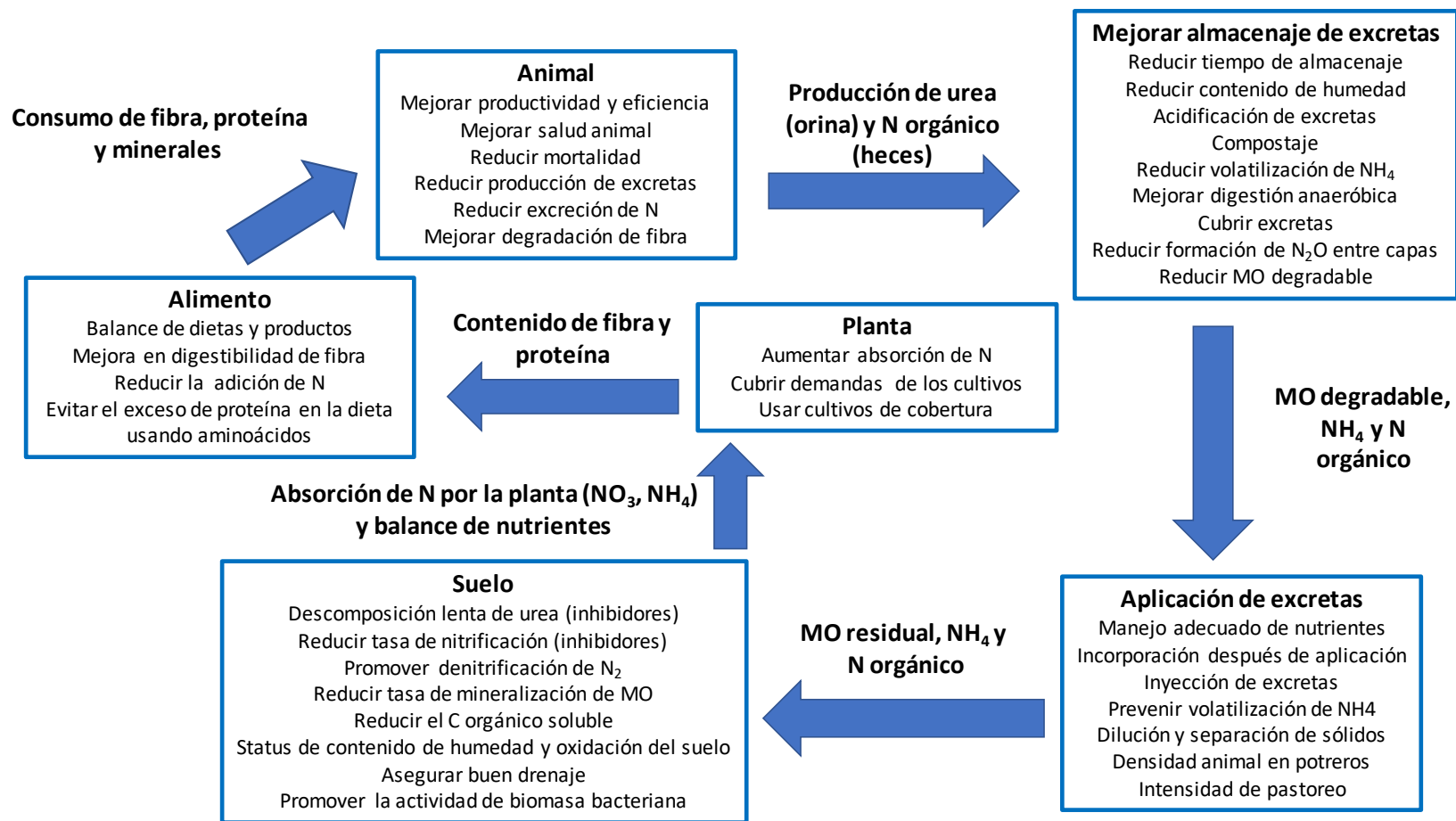
Figura 14. Oportunidades para mitigar el óxido nitroso de las excretas del ganado (Adaptado de: Montes et al. 2013).
