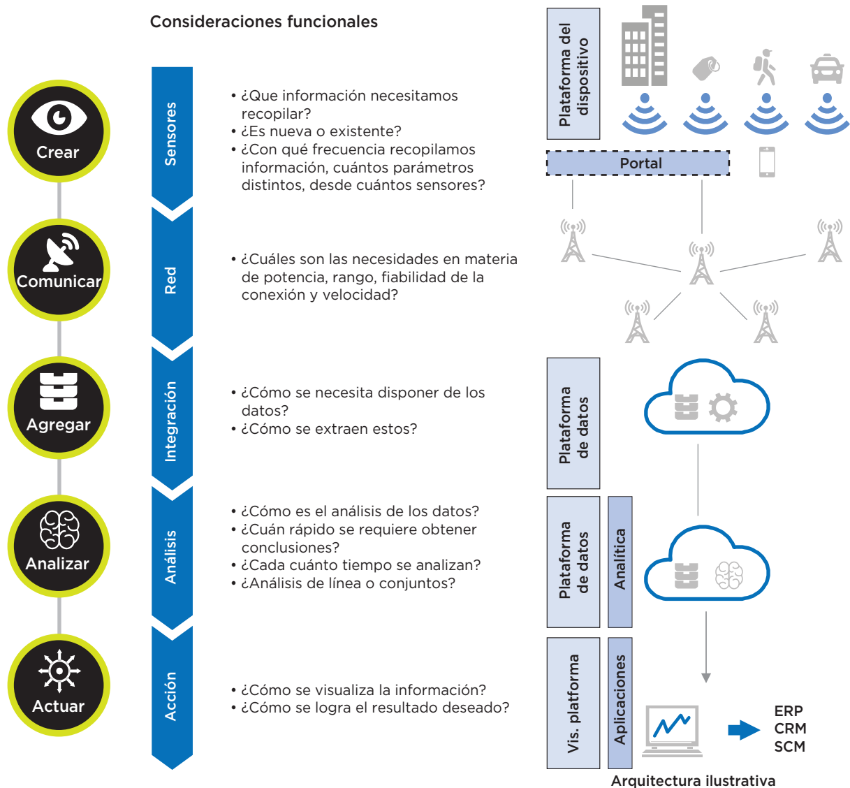
GRÁFICO 69 Arquitectura ilustrativa de redes de IoT
