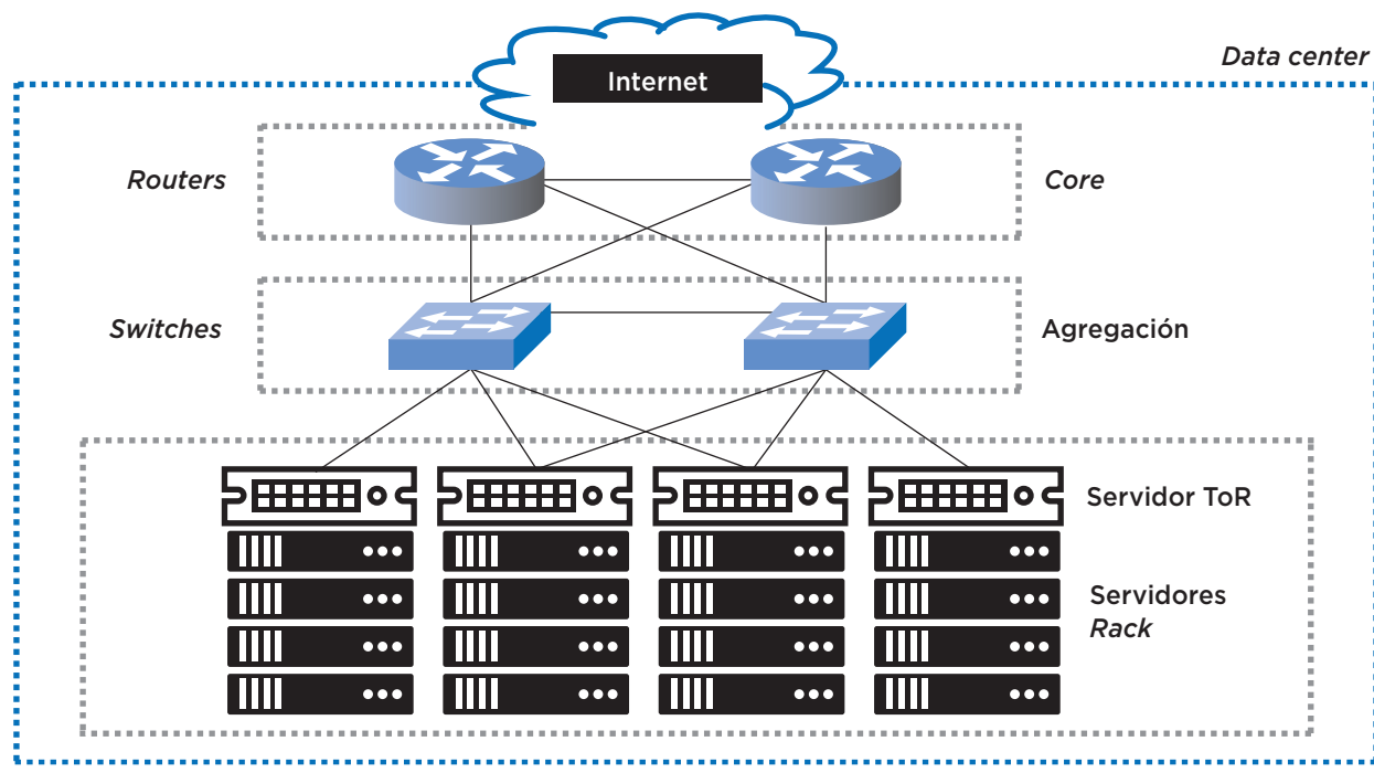
GRÁFICO 83 Infraestructura de un data center
